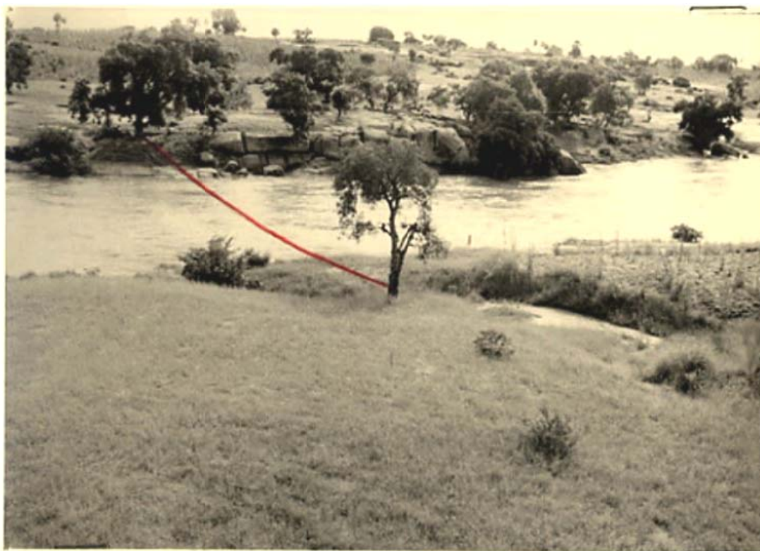
Goulbi de Maradi : Section de jaugeages de la station Nielloua Août 1957 © SIEREM
